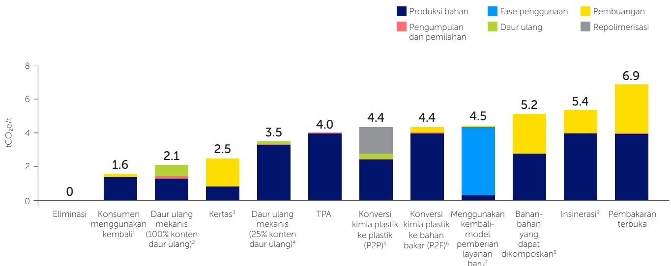
Gambar 10: Emisi gas rumah kaca dari 1 ton daya guna plastik Pilihan pengolahan yang berbeda memiliki dampak gas rumah kaca yang sangat berbeda
