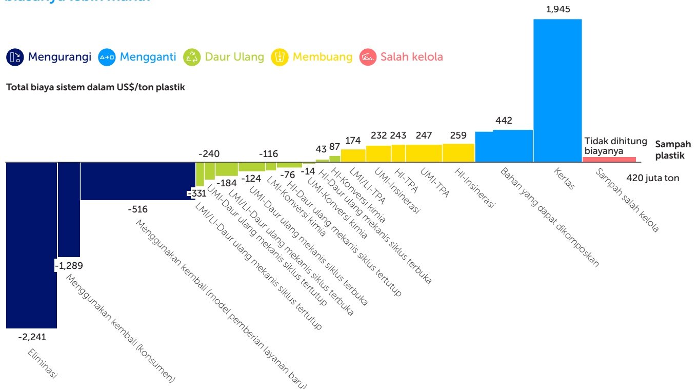
Gambar 13: Biaya dan jumlah per jenis pengolahan dalam Skenario Perubahan Sistem, 2040 Pengungkit Mengurangi seringkali paling ekonomis untuk diterapkan sedangkan pengganti plastik biasanya lebih mahal
